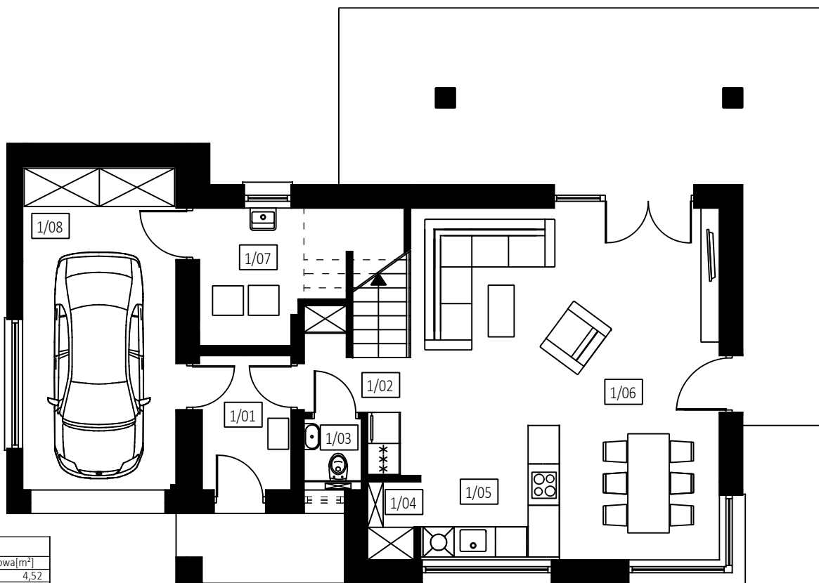
PARTER - zestawienie pomieszczeń
