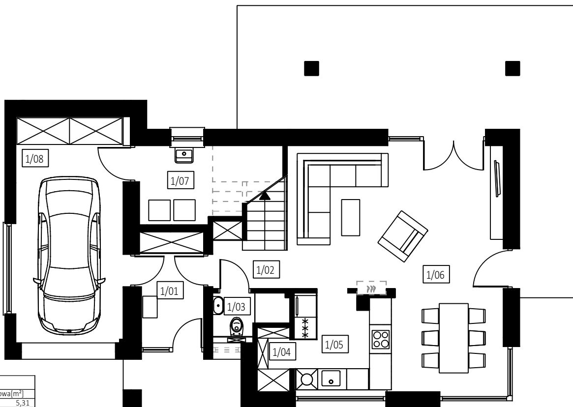
PARTER - zestawienie pomieszczeń
